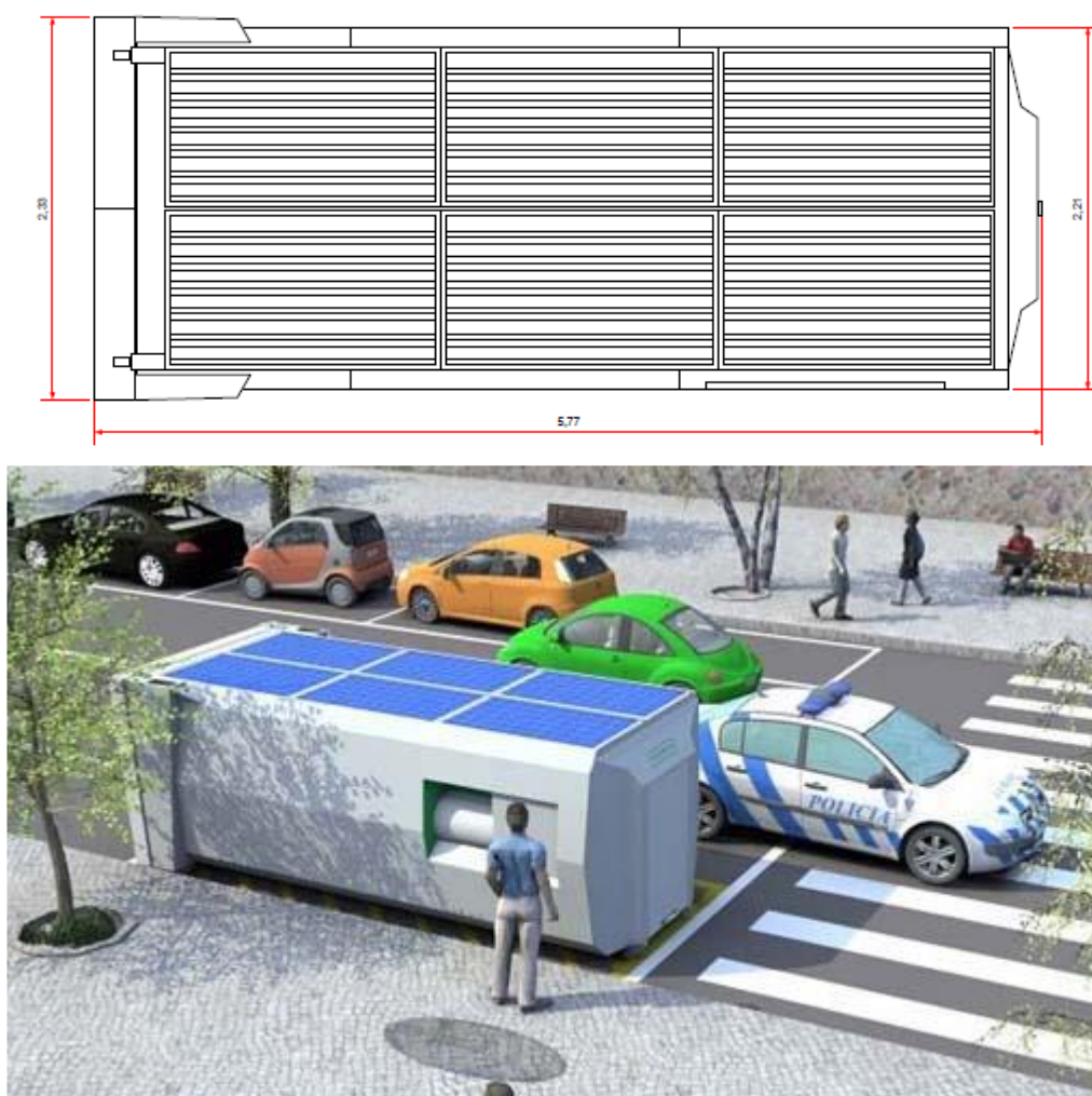
Εικόνα 19: Υπέργεια Γωνιά Ανακύκλωσης με ηλιακό συμπιεστή ανακύκλωσης
